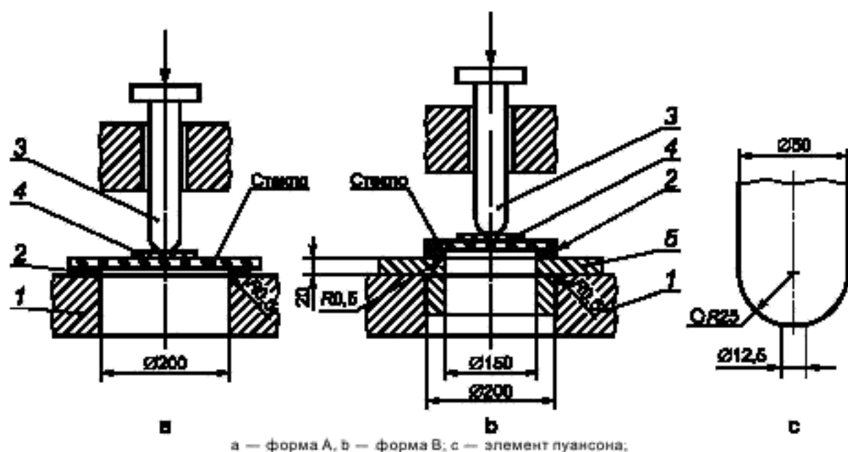
Рисунок 1 — Формы приспособлений
