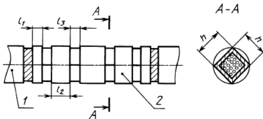
1 — кабель, 2 — гильза
