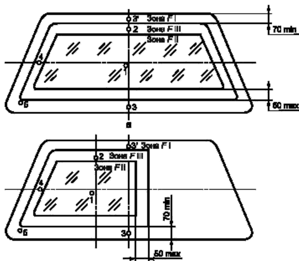
Рисунок 2 — Предписанные точки удара для ветровых стекол
