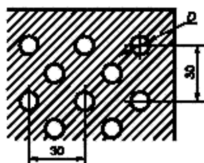
Рисунок 10 — Увеличенная деталь
