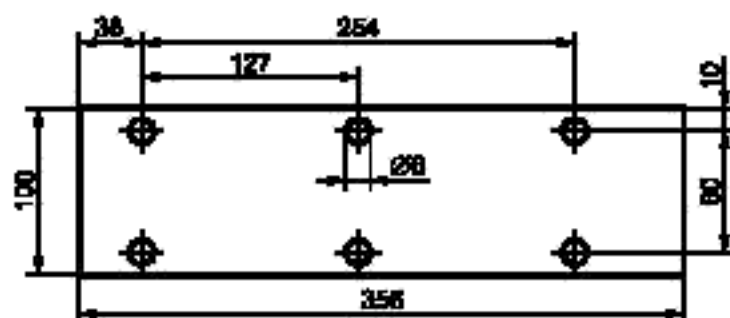
Рисунок 22 — Образец для испытаний
