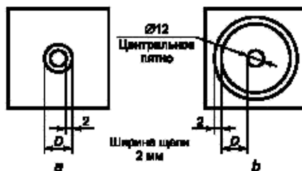
Рисунок 13 — Размеры мишеней
