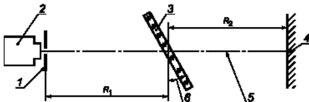
1 — диафрагма; 2 — проектор; 3 — безопасное стекло; 4 — проекционный экран; 5 — направление наблюдения; β — угол наклона; R_1 = 4 м; R_2 = 2-4 м (предпочтительно 4 м)
