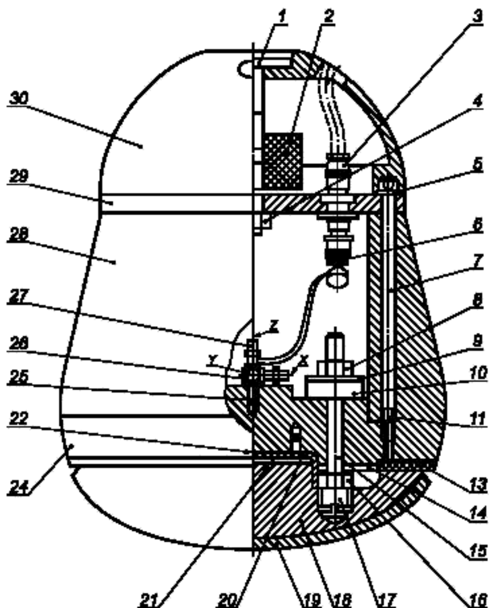
Рисунок 4 — Модель головы массой 10 кг
