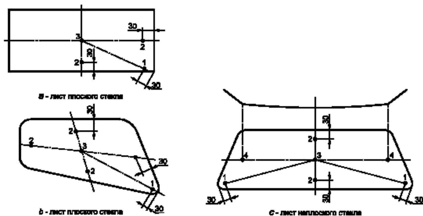
Рисунок 3 — Предписанные точки удара для равномерно упрочненных стекол
