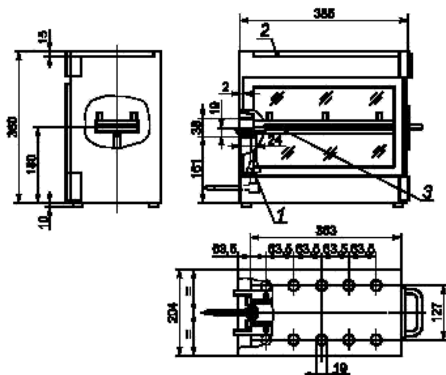
Рисунок 18 — Образец камеры сгорания
