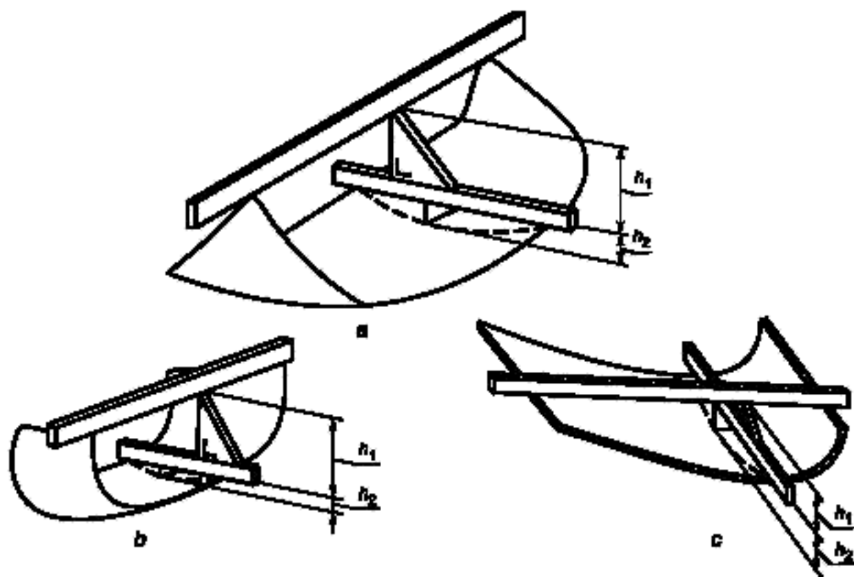
Рисунок 1 — Определение высоты сегмента h
