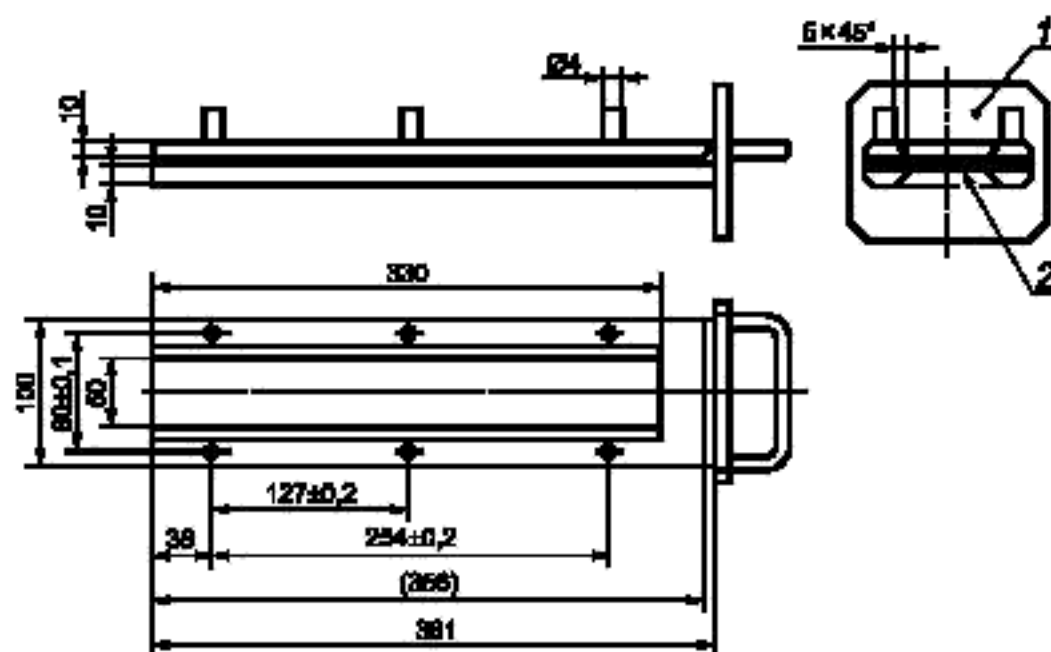
Рисунок 20 — Схема подставки
