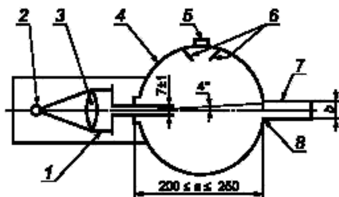
Рисунок 7 — Прибор для измерения уменьшения видимости
