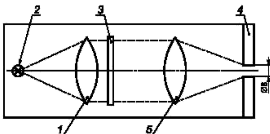
1 — конденсор; 2 — источник света; 3 — диапозитив (растр); 4 — диафрагма; 5 — линза
