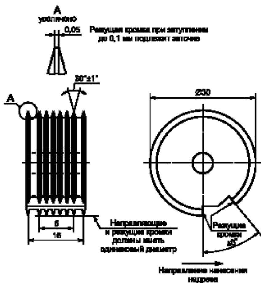
Рисунок 26 — Инструмент с шестью режущими элементами
