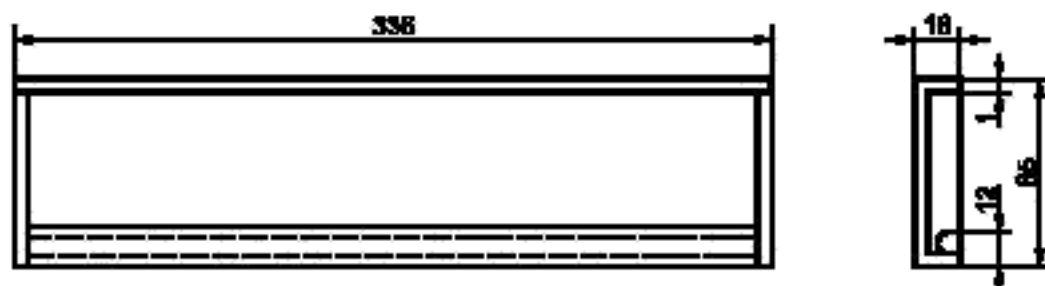
Рисунок 19 — Ванночка
