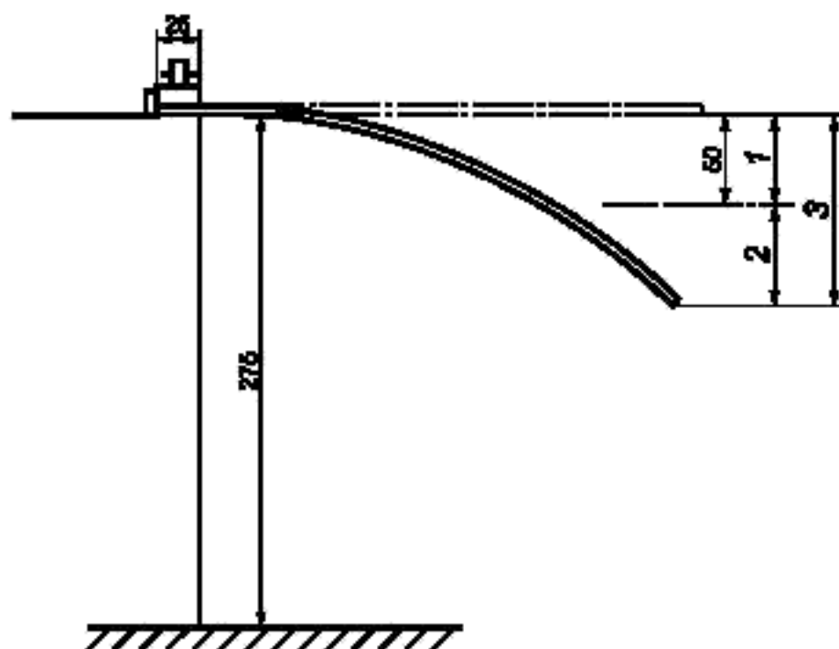
Рисунок 25 — Установка для испытания на гибкость
