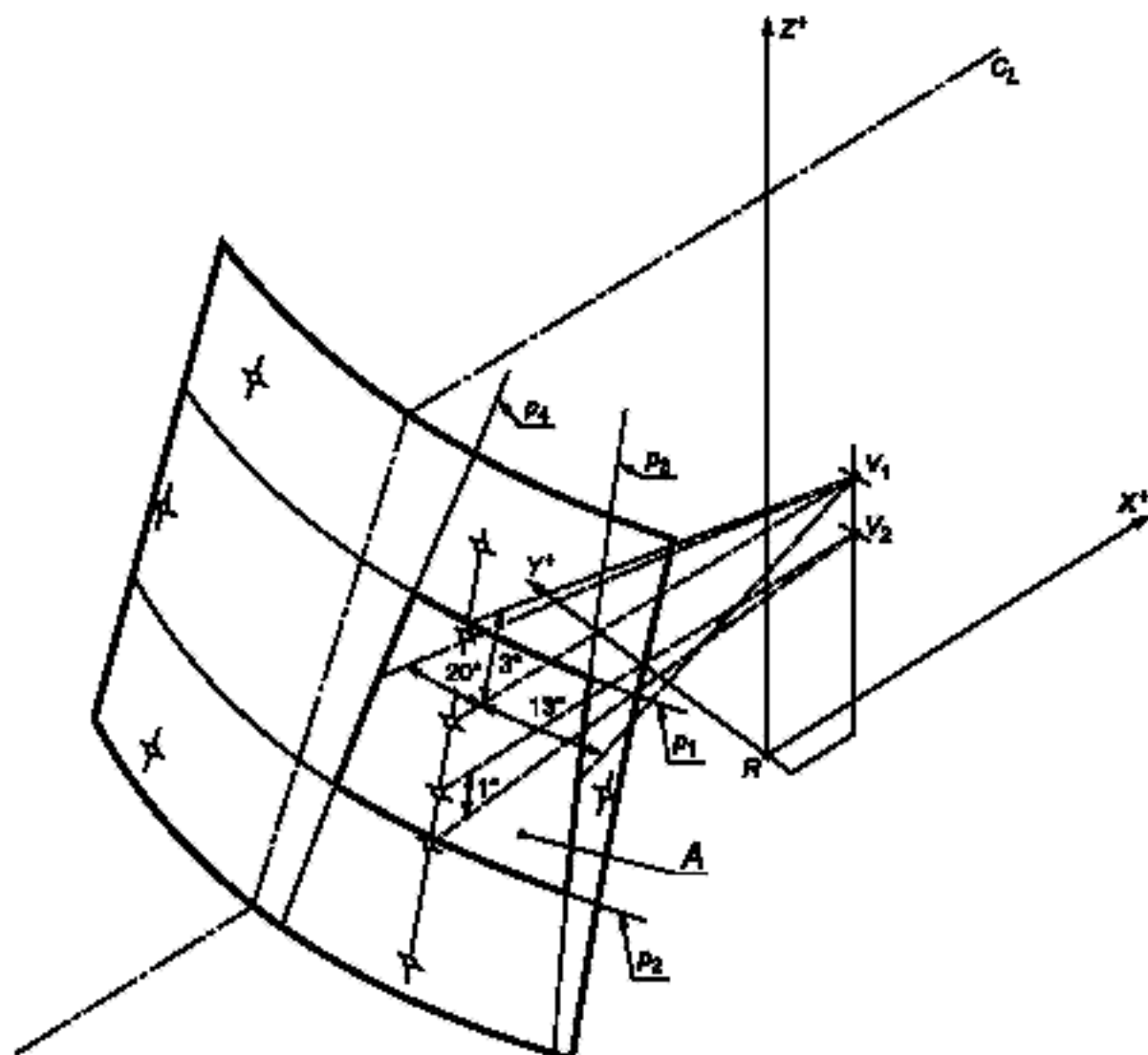
C_L — след продольного среднего сечения ТС; p — след соответствующей плоскости
