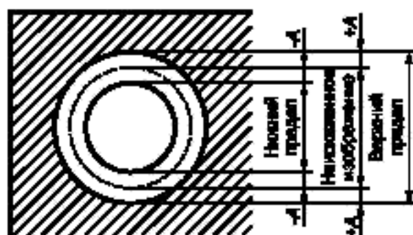
Рисунок 12 — Образец контрольного шаблона
