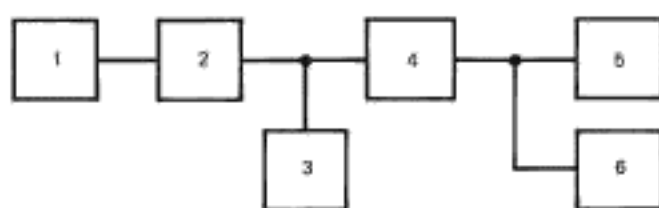
1 – измерительный компакт-диск (п. 2.2.14); 2 – измеряемый проигрыватель, 3 – эквивалент емкостной нагрузки (п. 2.2.16); 4 – фильтр верхних частот (п. 2.2.13); 5 – анализатор спектра (п. 2.2.5); 6 – вольтметр В2 (п. 2.2.4)
