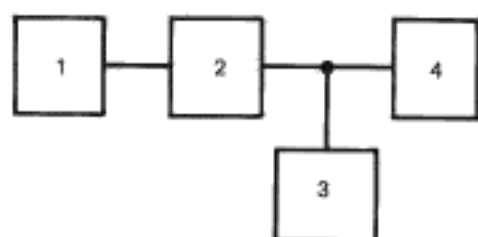
1 – измерительный компакт-диск (п. 2.2.14); 2 – измеряемый проигрыватель; 3 – эквива- лент резистивно-емкостной нагрузки (п. 2.2.15); 4 – вольтметр В2 (п. 2.2.4)
