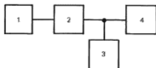
1 — измерительный компакт-диск (п. 2.2.14); 2 — измеряемый проигрыватель; 3 — эквивалент резистивно-емкостной нагрузки (п. 2.2.15); 4 — регистрирующее устройство (п. 2.2.2)
