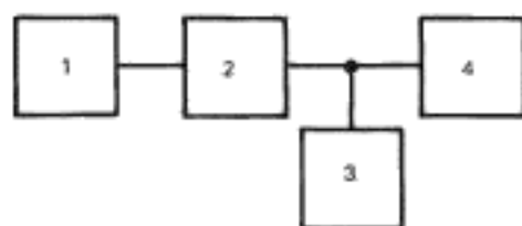
1 – измерительный компакт-диск (п. 2.2.14); 2 – измеряемый проигрыва- тель; 3 – эквивалент резистивно-емкостной нагрузки (п. 2.2.15); 4 – ана- лизатор спектра (п. 2.2.5)
