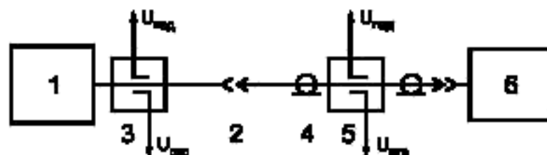
1 — передатчик; 2 — вход антенно-фидерного тракта (выход передатчика); 3 — рефлектометр на выходе передатчика; 4 — фидер антенны; 5 — рефлектометр, установленный в фидерном тракте антенны; 6 — антенна
