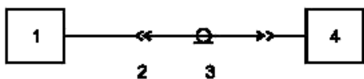
1 — измеритель КСВН; 2 — коаксиальный переход; 3 — фидер антенны; 4 — антенна
