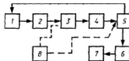
1 — анализатор боковых полос по 6.2.2; 2 — передатчик; 3 — согласованная нагрузка по 6.2.3; 4 — аттенюатор дополнительный; 5 — согласованный трюбник; 6 — демодулятор по 6.2.1; 7 — осциллограф по 6.2.6; 8 — направленный ответвитель по 6.2.4
