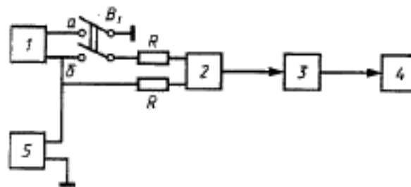
1 — генератор сигналов НЧ по 6.2.8; 2 — передатчик; 3 — эквивалент системы по 6.2.3; 4 — девиометр по 6.2.9; 5 — вольтметр НЧ по 6.2.10; R — измерительное сопротивление 300 \text{ Ом} \pm 0,2 \%
