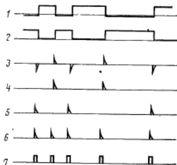
1—входной сигнал; 2—сигнал после формирователя; 3—сигнал на выходе дифференцирующей цепи; 4—неинвертируемые положительные импульсы; 5—сигнал на выходе инвертора; 6—сигнал на входе мультивибратора; 7—выходные импульсы
