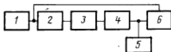
1—генератор сигналов НЧ; 2—датчик испытательных сигналов; 3—генератор сигнала ВЧ; 4—приемник; 5—эквивалент нагрузки; 6—измеритель краевых искажений
