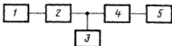
1—источник напряжения постоянного тока; 2—миллиамперметр постоянного тока; 3—вольтметр постоянного тока; 4—возбудитель; 5—эквивалент нагрузки
