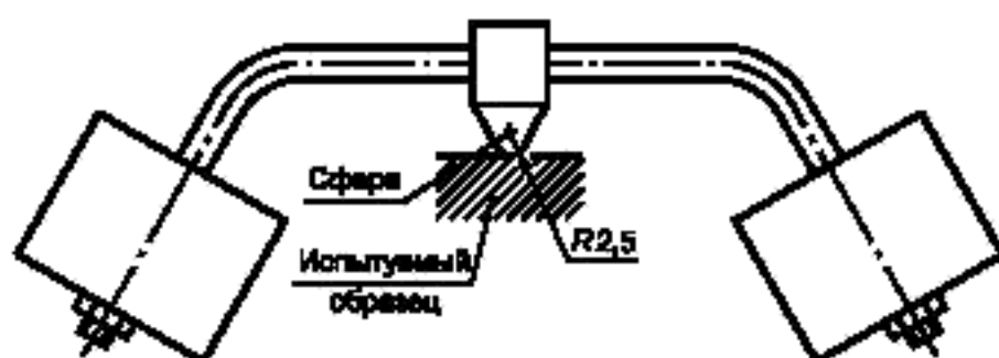
Рисунок 1 — Установка для испытания на теплостойкость
