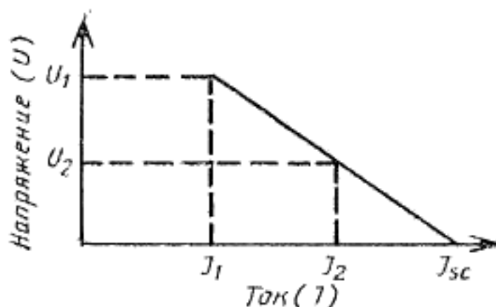
Рисунок 1 — Разрядная характеристика U=f(I)
