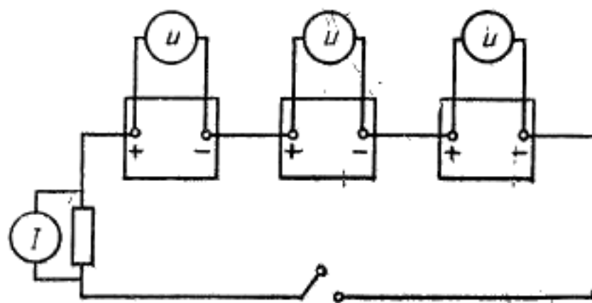
Рисунок 2 — Схема соединения
