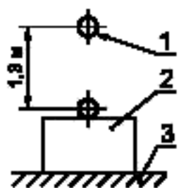
1 — стальной шарик; 2 — светильник; 3 — опорная поверхность
