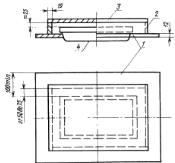
1 — основа, 2 — боковая стенка, 3 — верхняя стенка, 4 — испытуемый светильник
