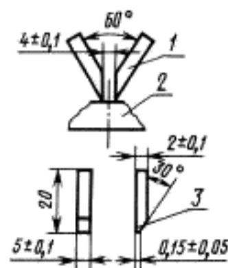
1 — электрод; 2 — испытуемый образец; 3 — конец электрода скручен Черт. 4
