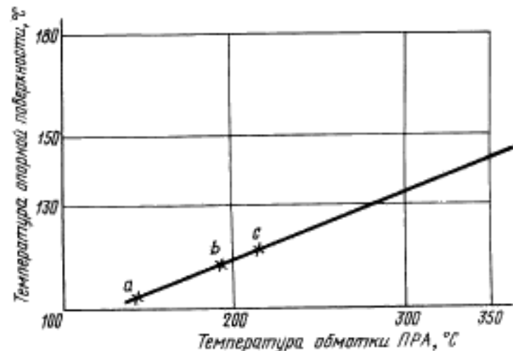
а, б, с — измеренные значения температуры при 0,9-, 1,0 и 1,1-кратном номинальном напряжении
