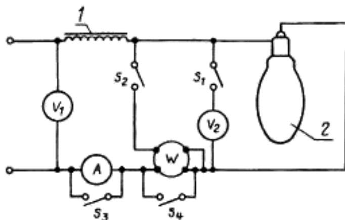
1 — образцовый балласт; 2 — лампа
