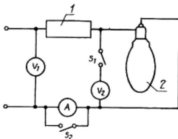
1 — балласт, 2 — лампа
