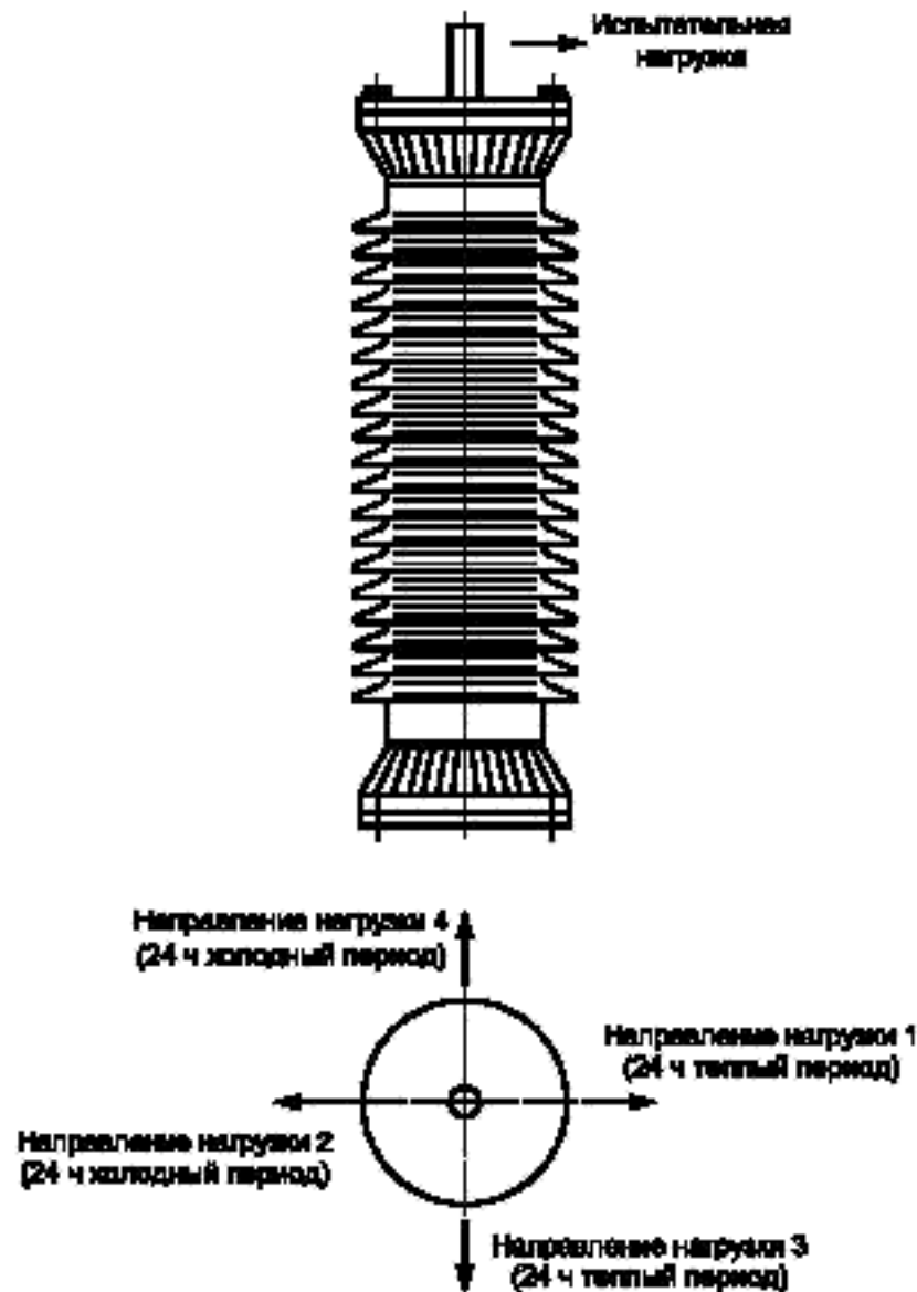
Рисунок 5 — Направления действия изгибающей нагрузки при термомеханических испытаниях
