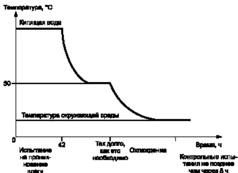
Рисунок 6 — Испытания на проникновение влаги
