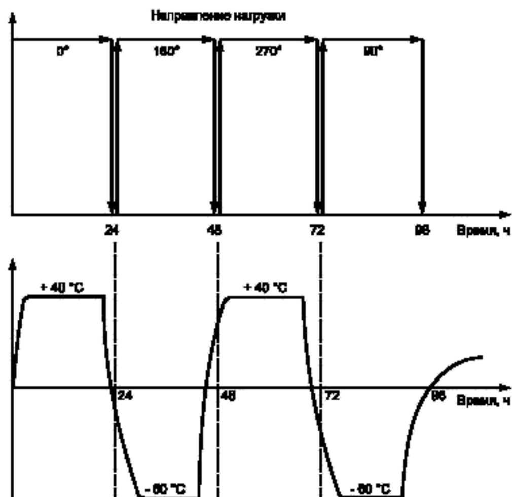
Рисунок 4 — Термомеханические испытания
