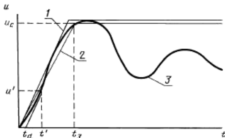
Построение огибающей ПВН, определяемого двумя параметрами
