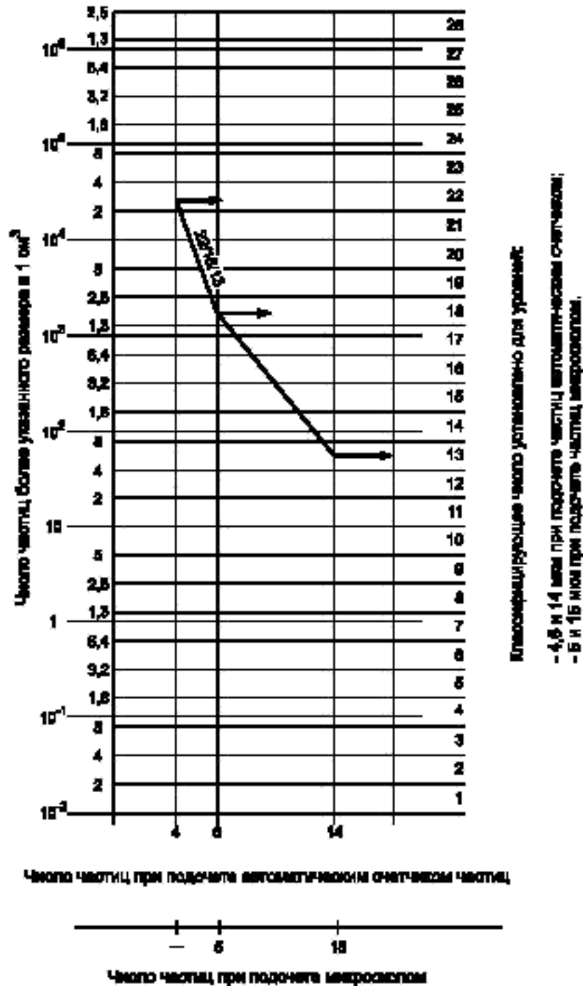
Рисунок Б.1 — Графическое представление кодового числа
