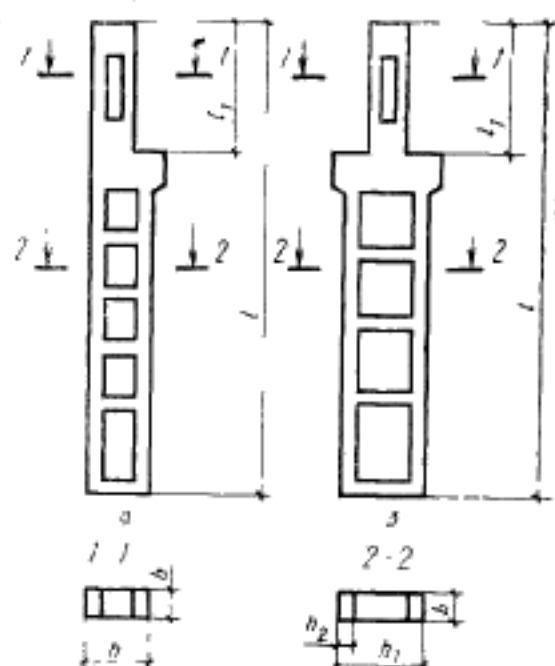
а—колонна крайних рядов; б—колонна средних рядов
