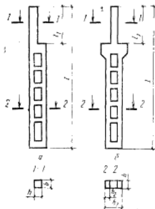
а—колонна крайних рядов; б—колонна средних рядов
