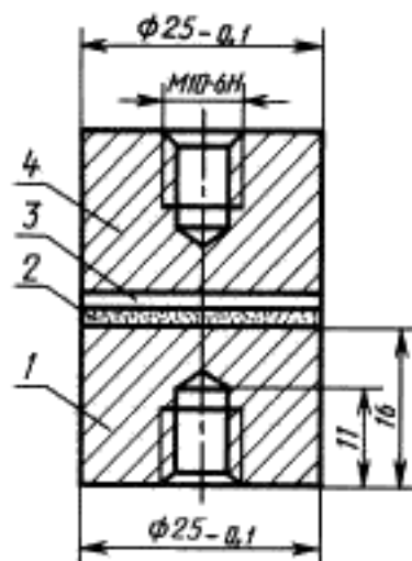
1 — образец; 2 — покрытие; 3 — клеевая прослойка; 4 — контробразец
