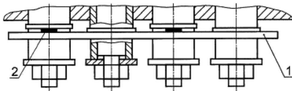
1 — поверочная линейка; 2 — щуп
