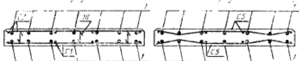
1 — напрягаемая арматура; 2 — крепление сеток С3
