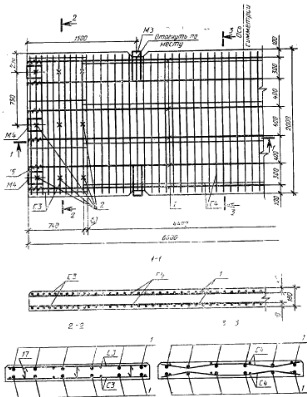
1 — напрягаемая арматура; 2 — крепление сеток С3
