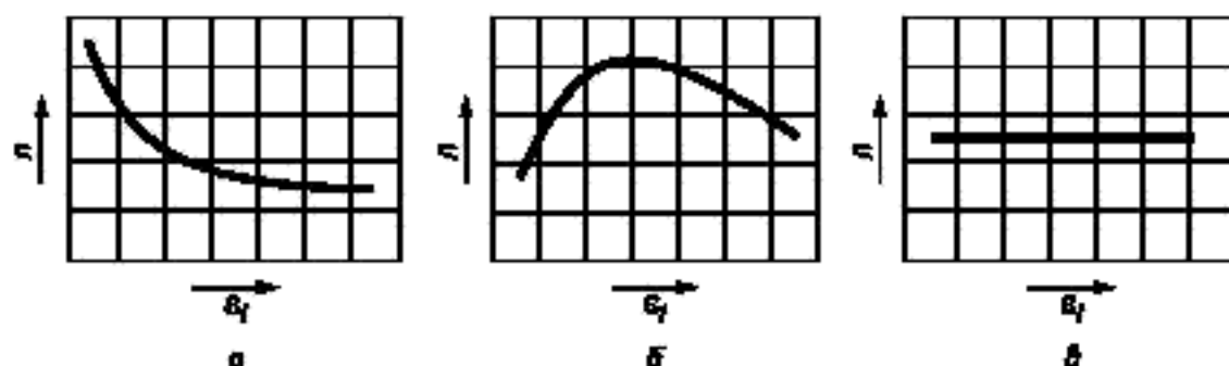
Рисунок Е.1 — Типовые зависимости показателя деформационного упрочнения n от степени деформации \epsilon_f
