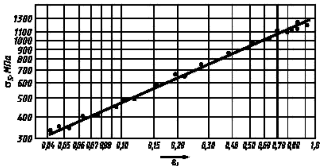
Рисунок 10 — Экспериментальная кривая упрочнения в логарифмических координатах
