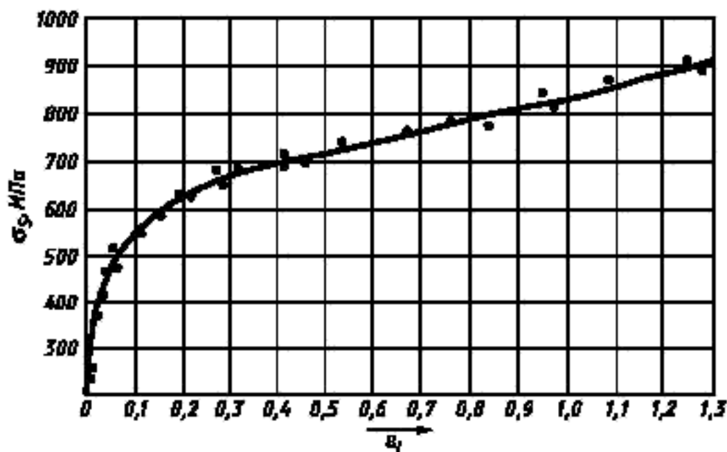
Рисунок 9 — Экспериментальная кривая упрочнения в координатах \sigma_t - \epsilon_t
