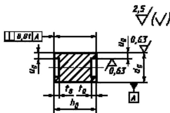
Рисунок 2 — Экспериментальные образцы IV типа
