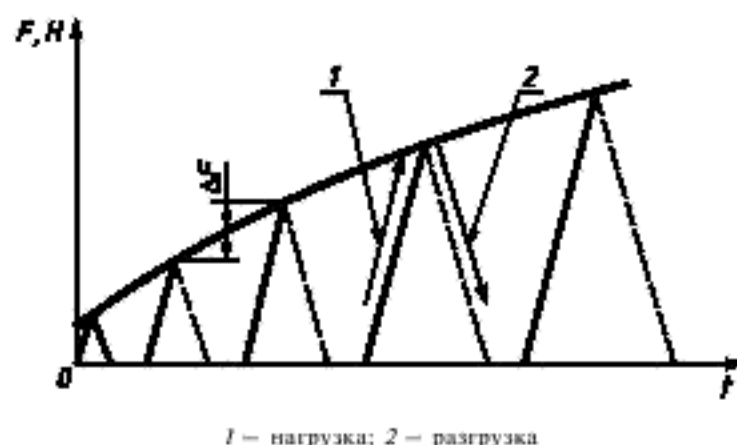
Рисунок 11 — Проведение испытаний при ступенчатом увеличении нагрузки
