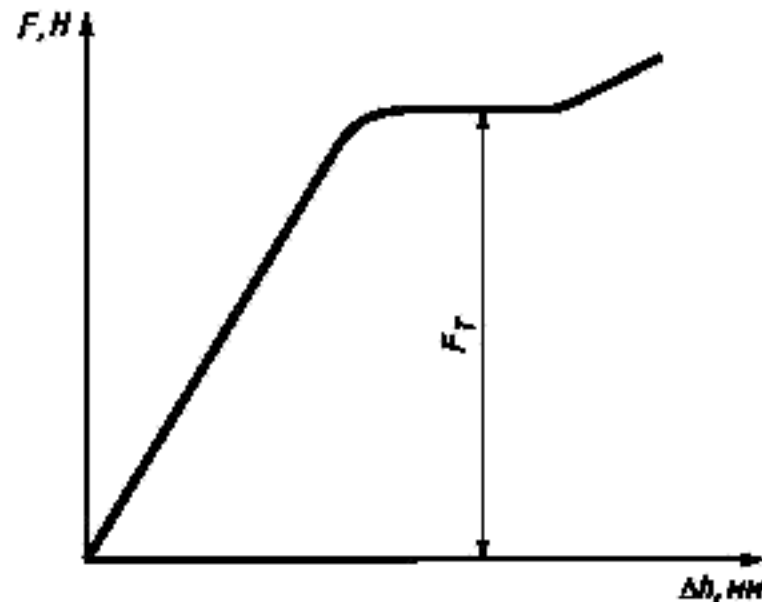
Рисунок 6 — Определение нагрузки F_{\tau} , соответствующей пределу текучести при сжатии
