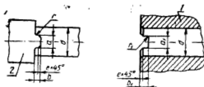
1 — инструмент; 2 — оправка
