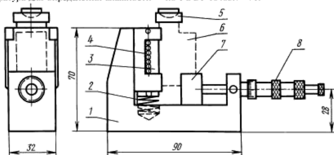
1 — корпус; 2 — пружина; 3 — подвижная планка; 4 — ролики; 5 — нажимная призма с шаровой опорой; 6 — образец; 7 — подвижная опора; 8 — устройство для прижима подвижной опоры Черт. 1
