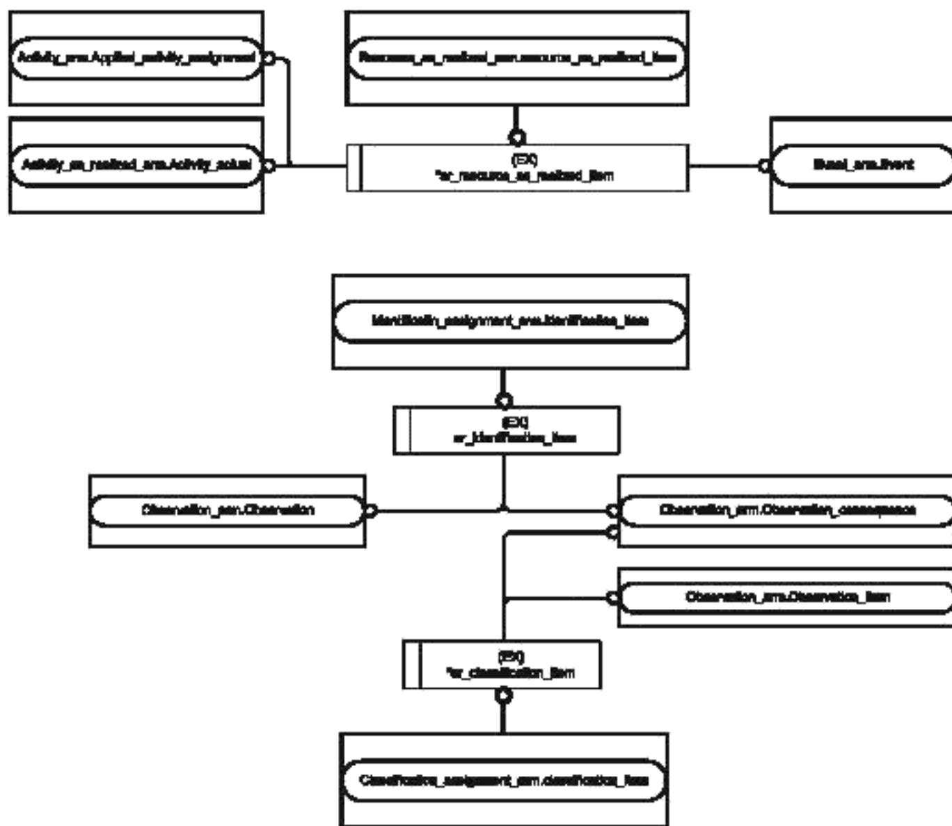
Рисунок С.3 — Представление ПЭМ на уровне объектов в формате EXPRESS-G (диаграмма 2 из 4)
