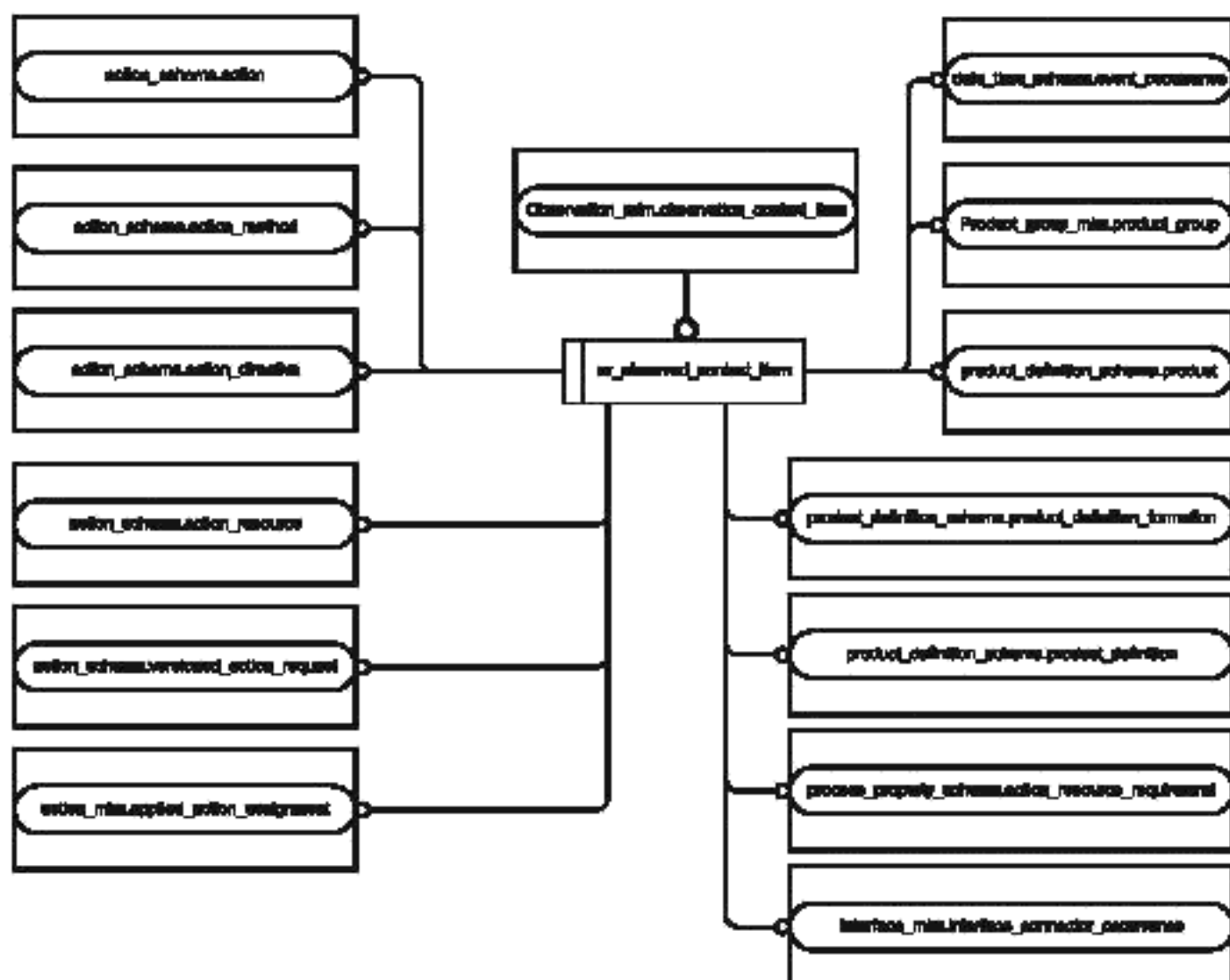
Рисунок D.5 — Представление IMM на уровне объектов в формате EXPRESS-G (диаграмма 4 из 4)
