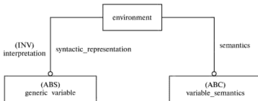
Рисунок D.1 — Связь синтаксиса и семантики переменной
