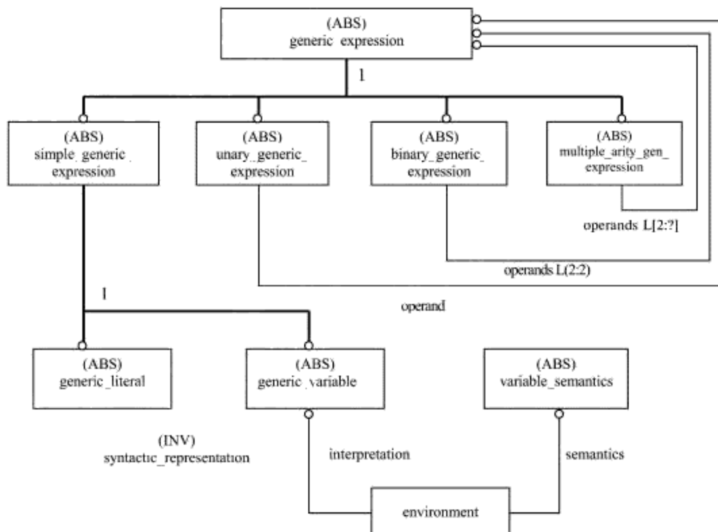
Рисунок С.1 — ISO13584_generic_expressions_schema — EXPRESS-G диаграмма 1 из 1
