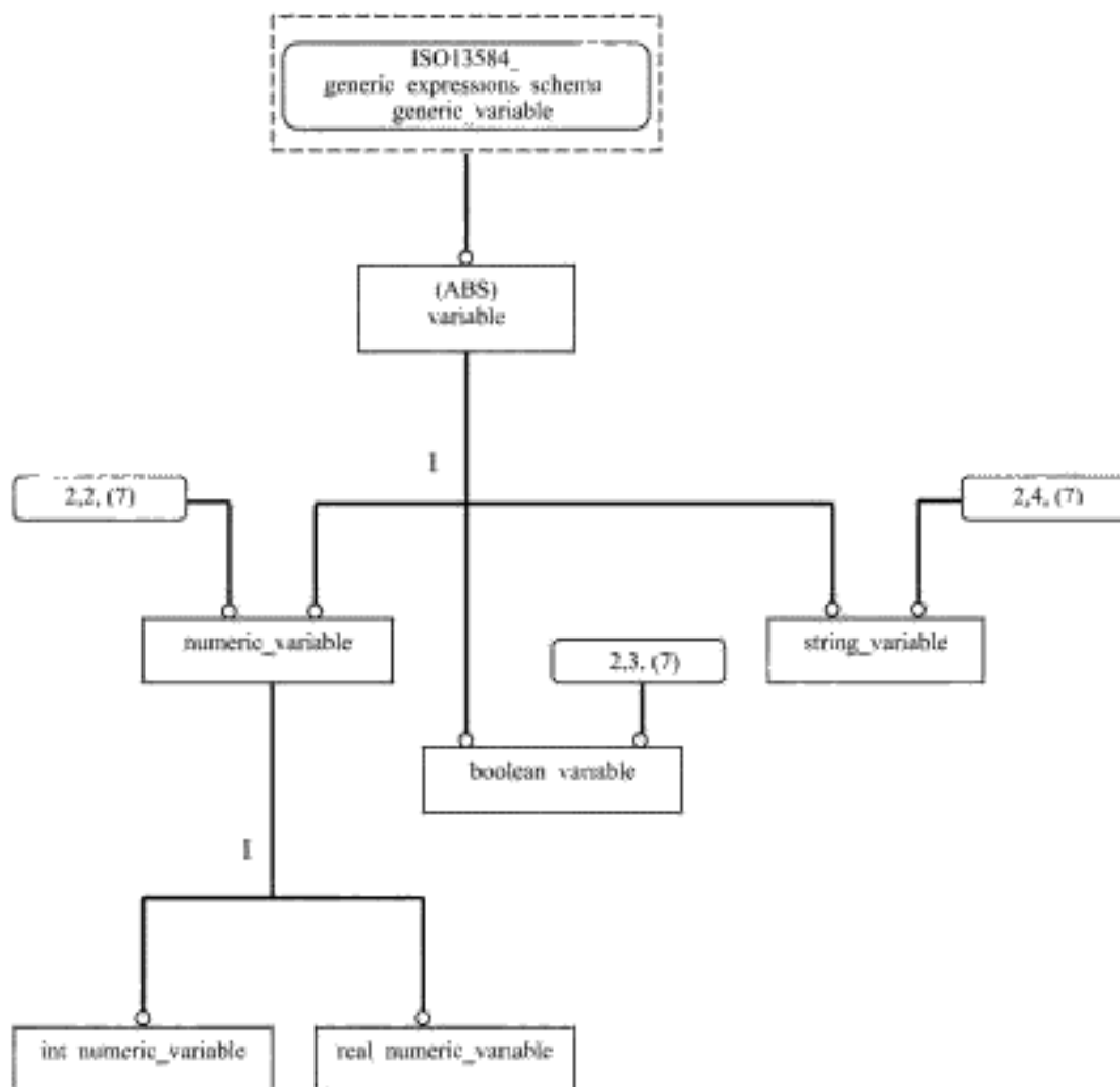
Рисунок С.3 — ISO13584_expressions_schema — EXPRESS-G диаграмма 2 из 12. Переменные
