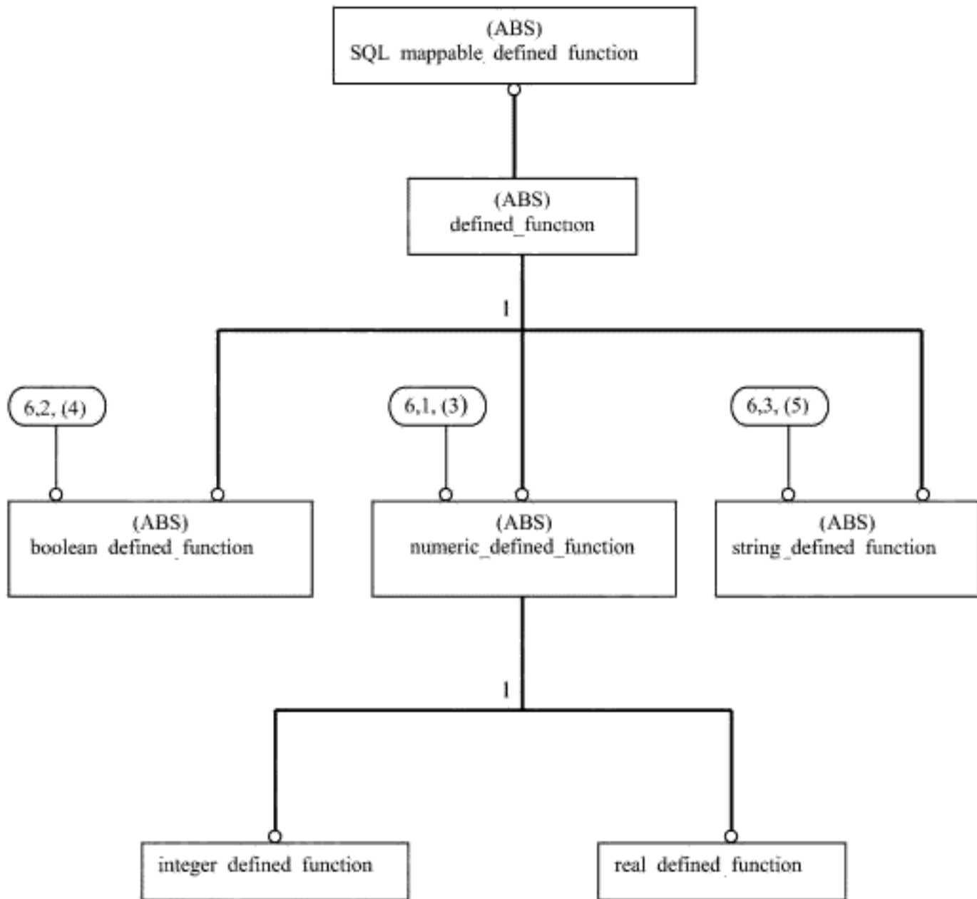
Рисунок С.7 — ISO13584_expressions_schema — EXPRESS-G диаграмма 6 из 12. defined_function
