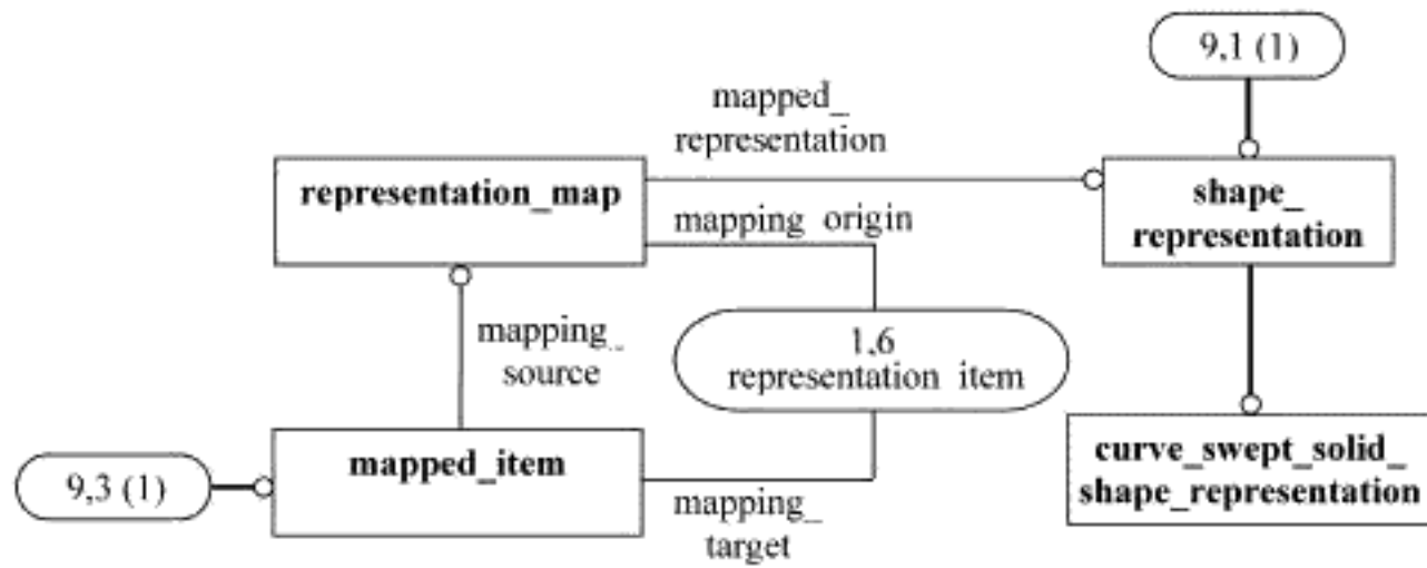
Рисунок D.9 — ПИК a1c_curve_swept_solid в формате EXPRESS-G (диаграмма 9 из 9)
