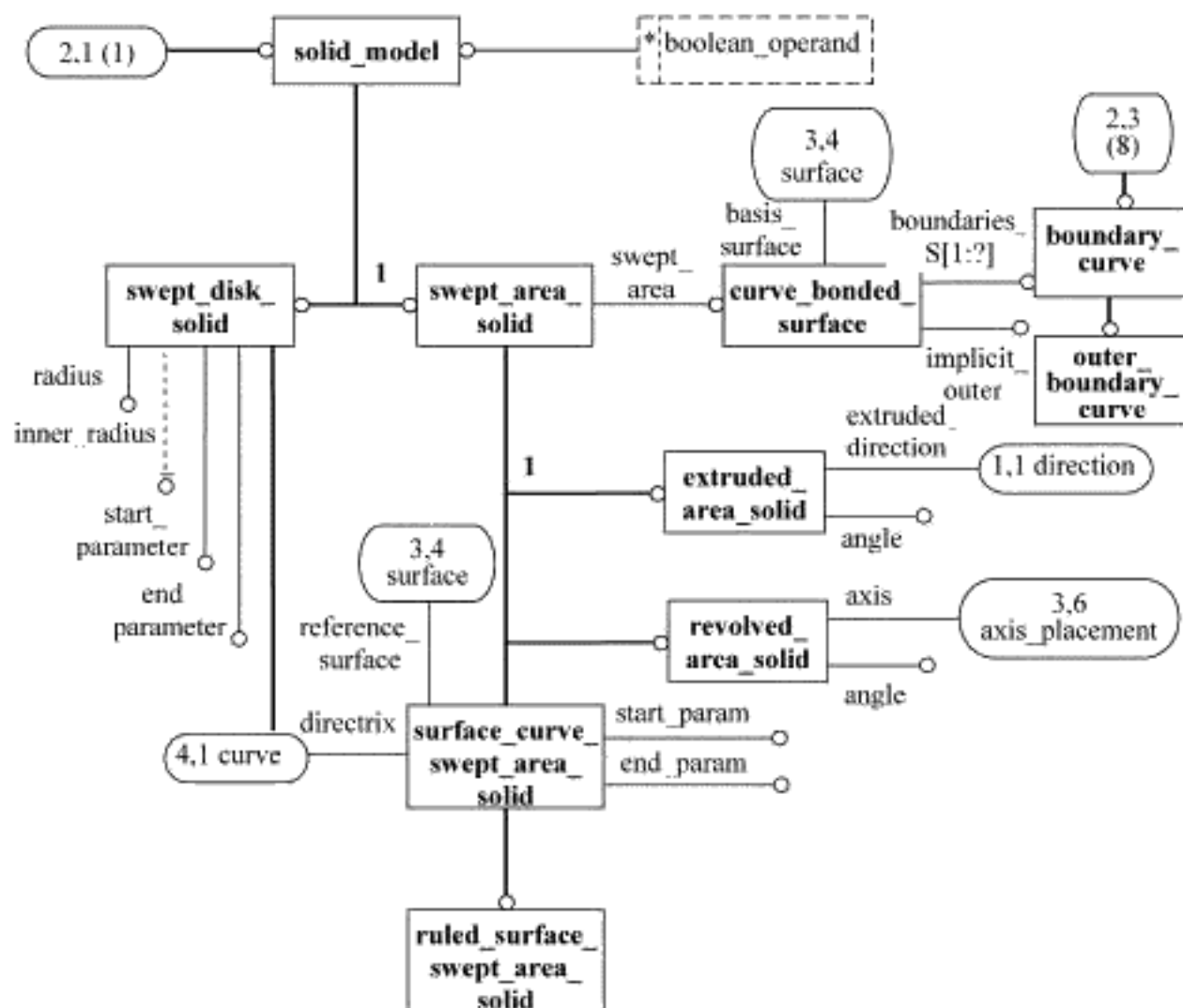
Рисунок D.2 — ПИК ais_curve_swept_solid в формате EXPRESS-G (диаграмма 2 из 9)
