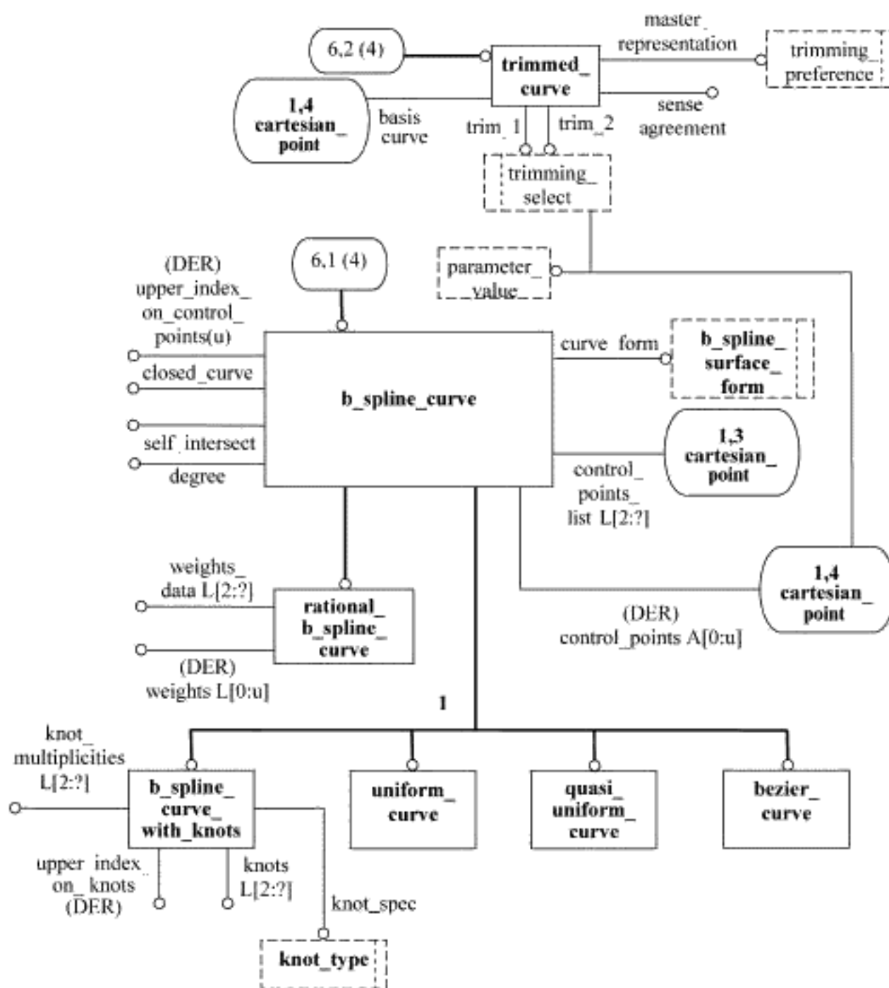
Рисунок D.6 — ПИК aic_curve_swept_solid в формате EXPRESS-G (диаграмма 6 из 9)
