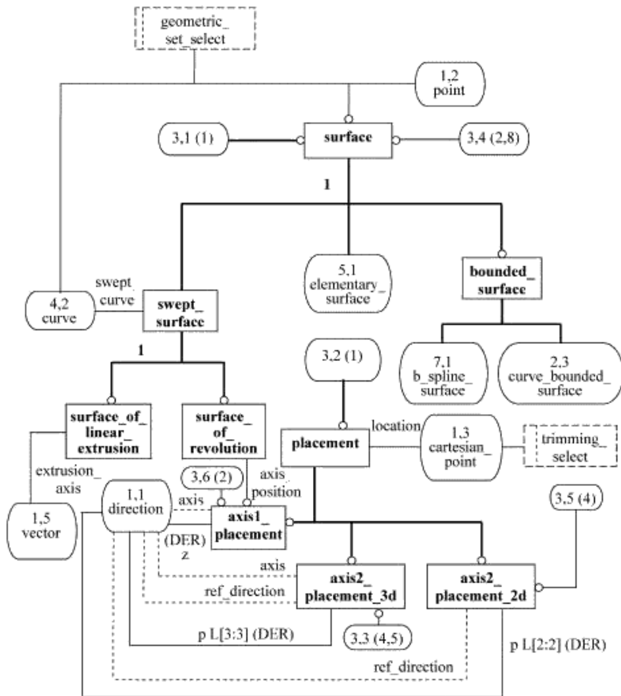
Рисунок D.3 — ПИК aic_curve_swept_solid в формате EXPRESS-G (диаграмма 3 из 9)
