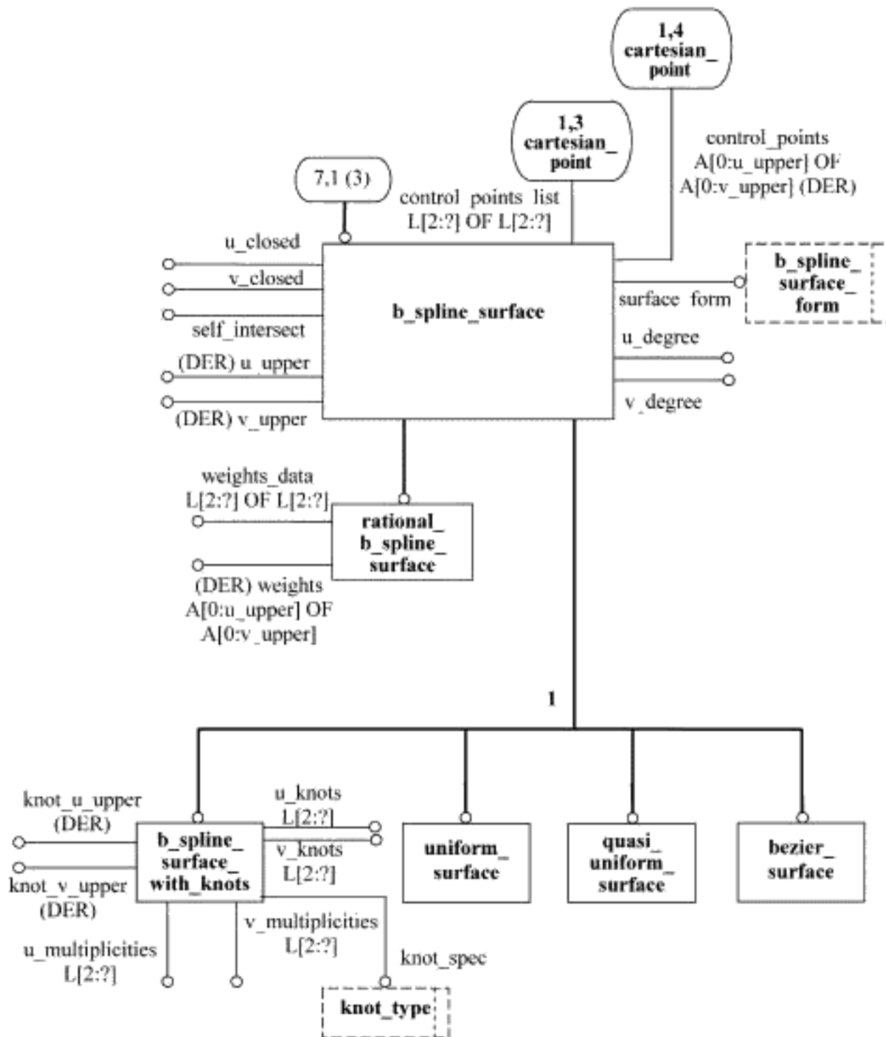
Рисунок D.7 — ПИК ais_curve_swept_solid в формате EXPRESS-G (диаграмма 7 из 9)
