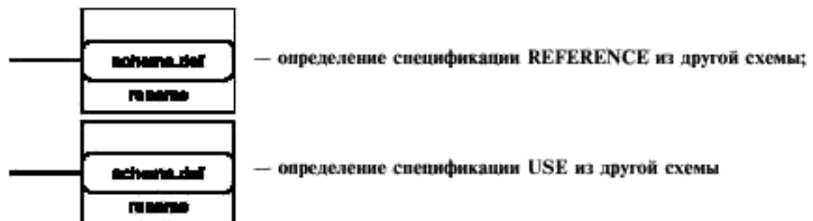
Рисунок D.13 — Символы компоновки: ссылки между схемами
