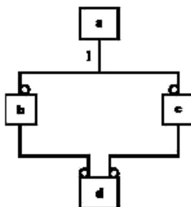
Рисунок В.2 — EXPRESS-G-диаграмма для схемы из примера 156
