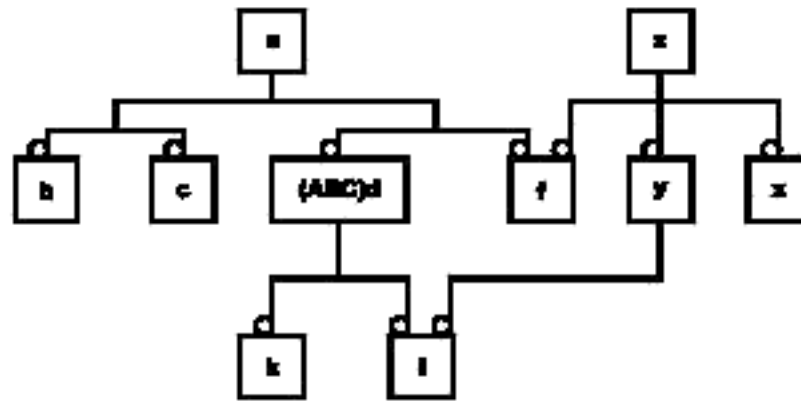
Рисунок В.3 — EXPRESS-G-диаграмма для схемы из примера 157
