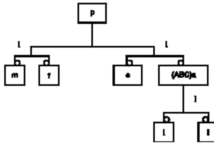
Рисунок В.1 — EXPRESS-G-диаграмма для схемы из примера 155
