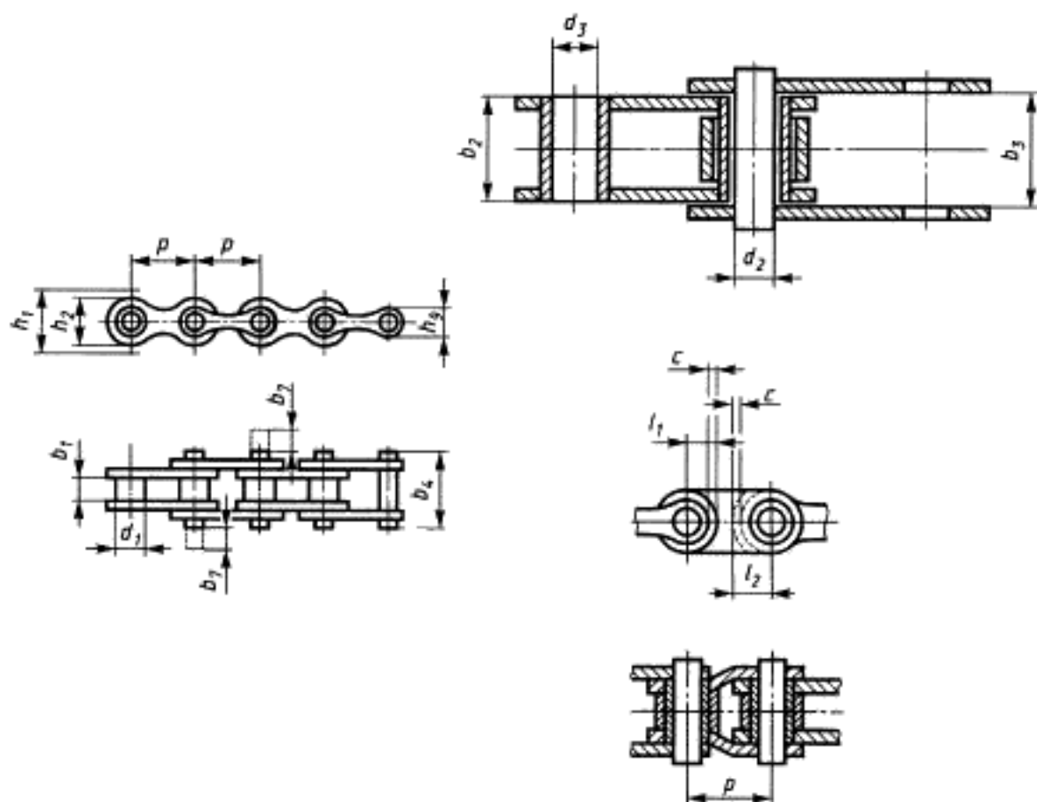
Рисунок 1 — Цепь
