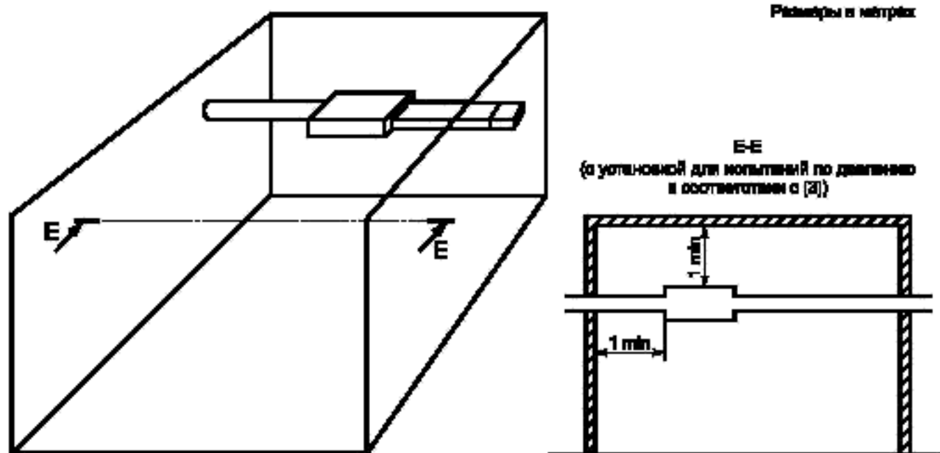
Рисунок 6 — Установка воздухораспределительного элемента для определения шума корпуса
