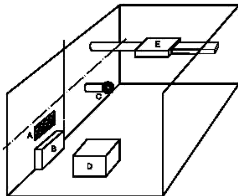
Рисунок 1 — Размещение оборудования в испытательном помещении
