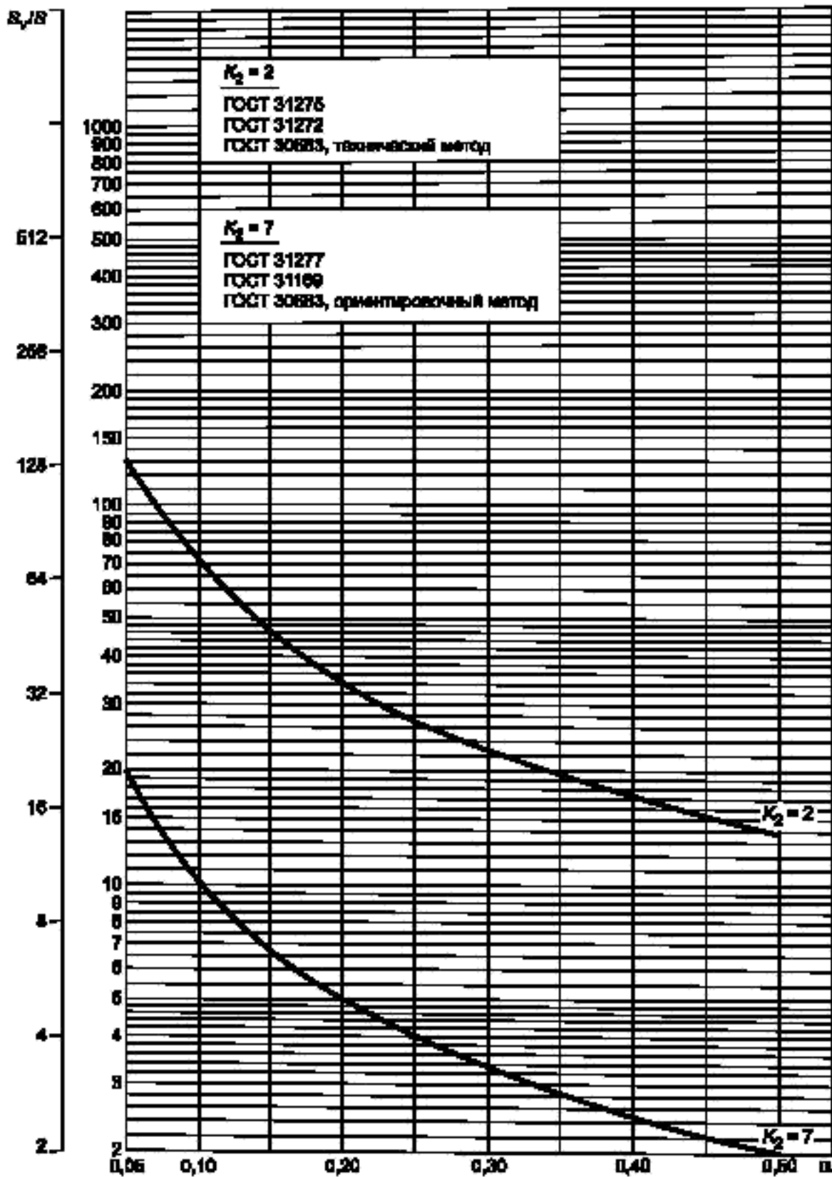
Рисунок С.1 — Значения \alpha и S_v/S
