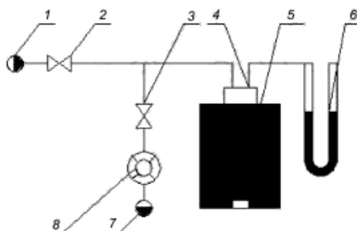
1 — устройство подачи воздуха; 2,3 — регулирующие вентили; 4 — соединительное устройство; 5 — аппарат; 6 — мановакуумметр; 7 — источник разрежения; 8 — газовый счетчик
