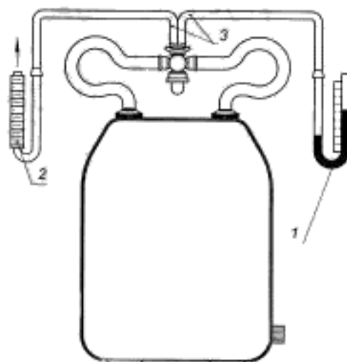
1 — мановакуумметр; 2 — ротаметр; 3 — соединительные трубки
