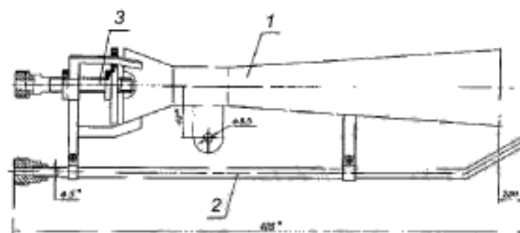
1 — диффузор, 2 — трубка поджига, 3 — сопло
