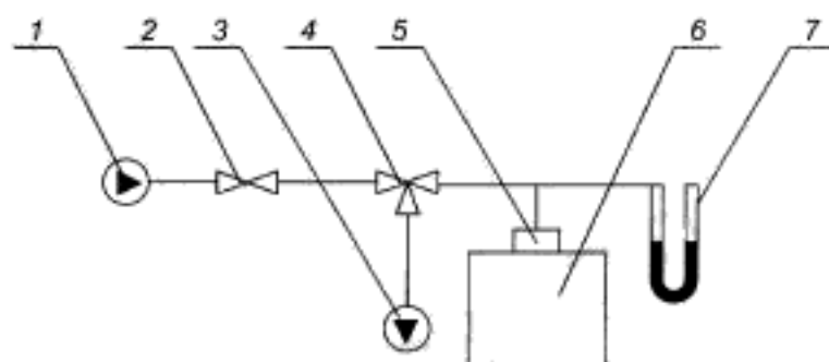
1 — источник давления; 2 — регулирующий вентиль; 3 — источник разрежения; 4 — трехходовой кран; 5 — соединительное устройство; 6 — аппарат; 7 — мановакуумметр
