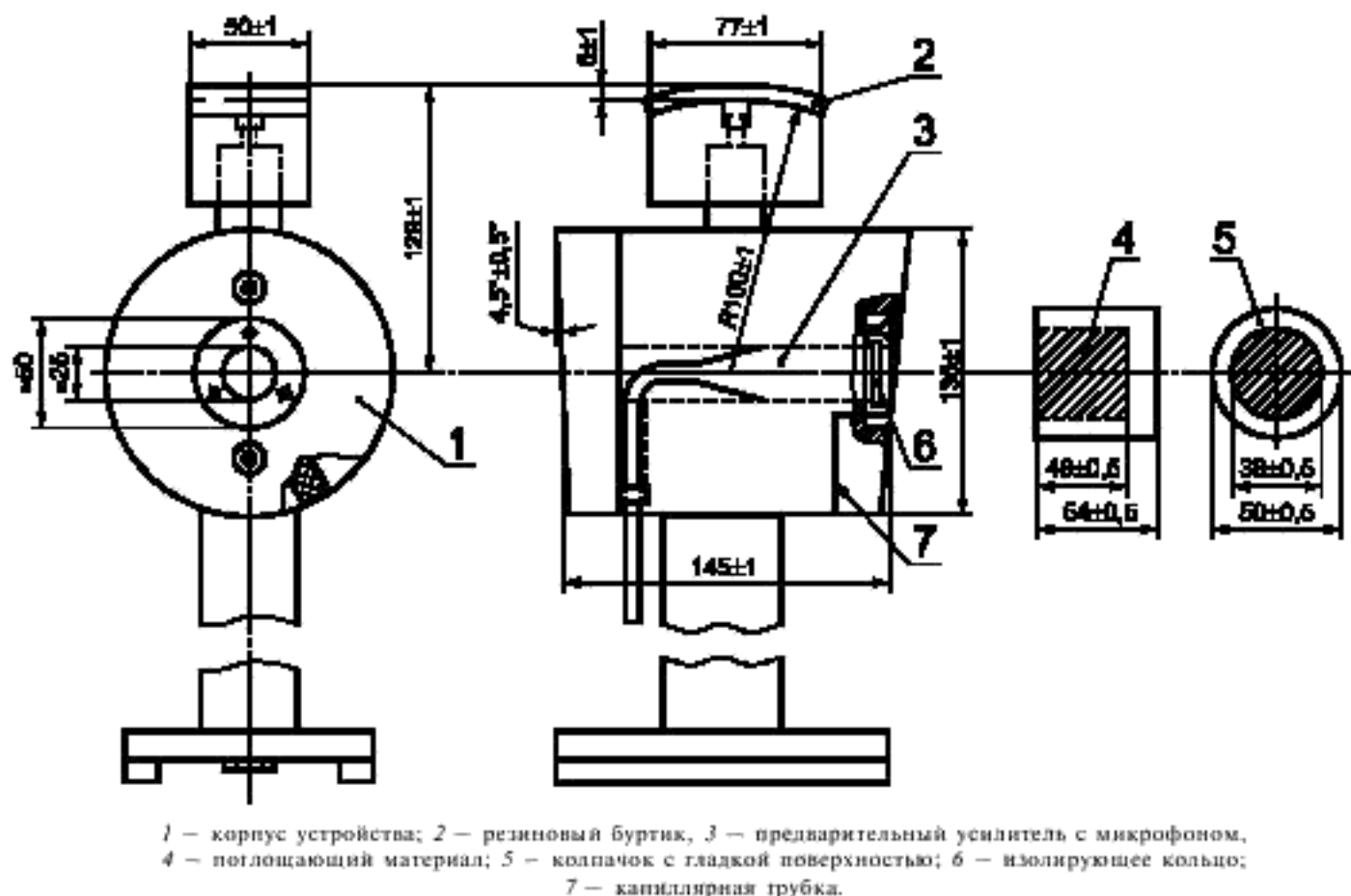
Рисунок 1 — Образец устройства для проведения акустического испытания
