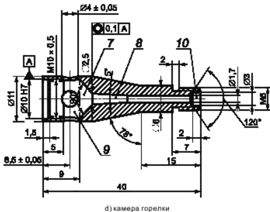
Рисунок 2 — Газовая горелка, лист 1
