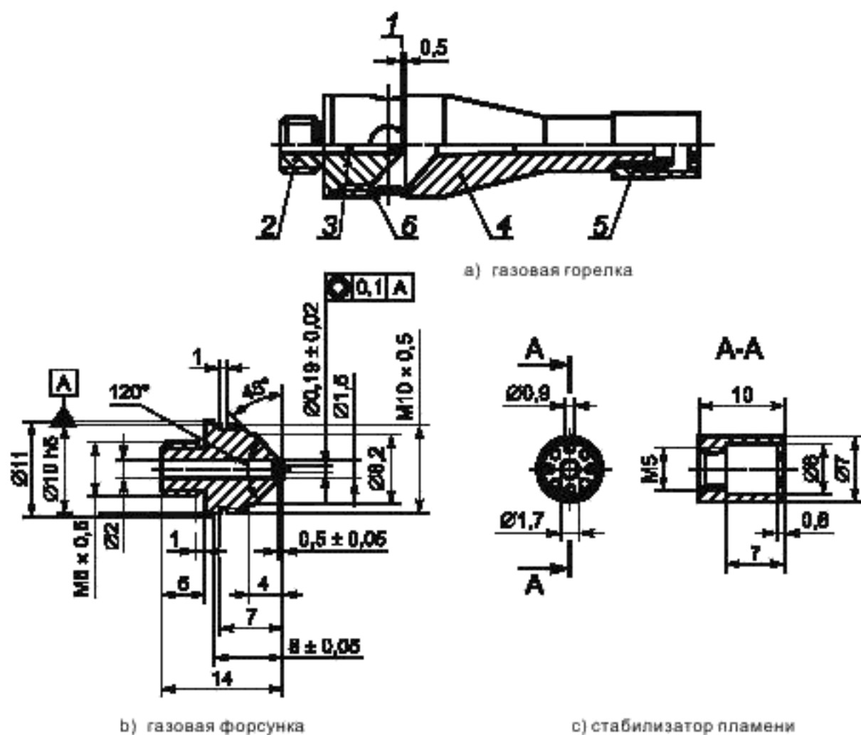
Рисунок 2 — Газовая горелка, лист 1
