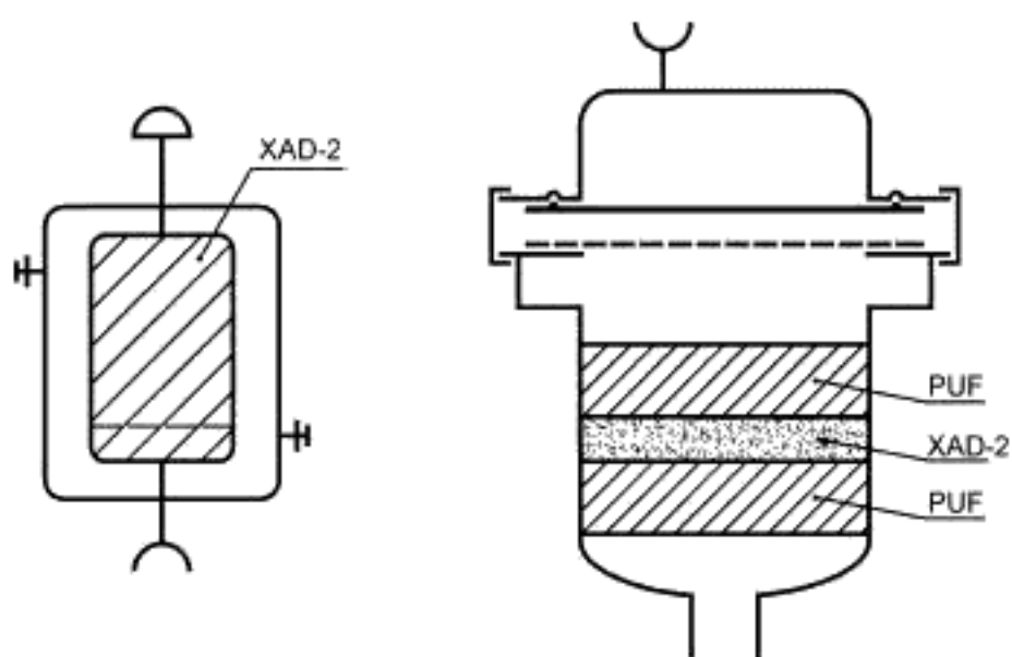
Рисунок В.6 — Схемы двух картриджей с сорбентом
