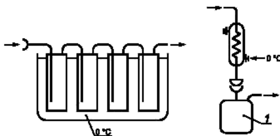
Рисунок В.5 — Схемы двух охлаждающих систем
