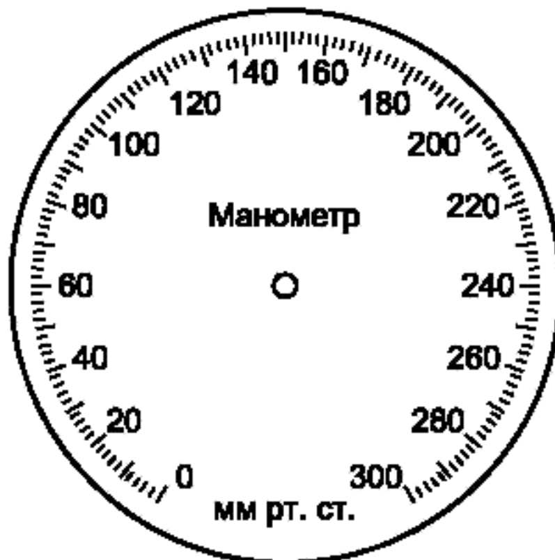
Рисунок 1 — Пример шкалы anerоидного манометра (деление, мм рт. ст., без поля допуска в положении нуля, см. 7.1.4.2.3)
