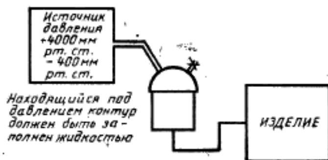
Рисунок 107 — Испытание давления, наращаемого постепенно (см. 45.101)
