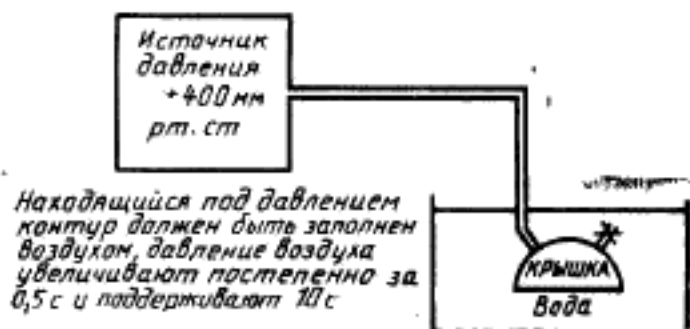
Рисунок 106 — Испытание герметичности диафрагмы (см. 17.101.2)
