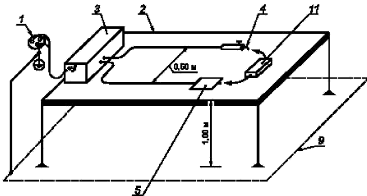
Рисунок 105 — Измерение ВЫХОДНОЙ МОЩНОСТИ. Монополярный выход (пункт 50)
