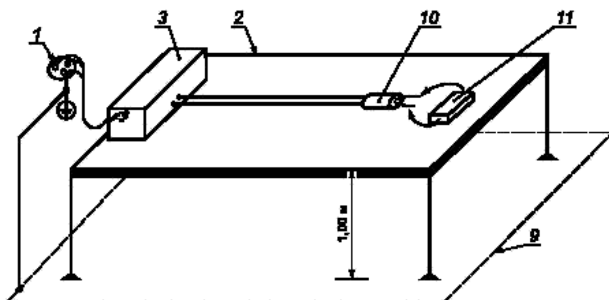
Рисунок 106 — Измерение ВЫХОДНОЙ МОЩНОСТИ. Биполярный выход (пункт 50)
