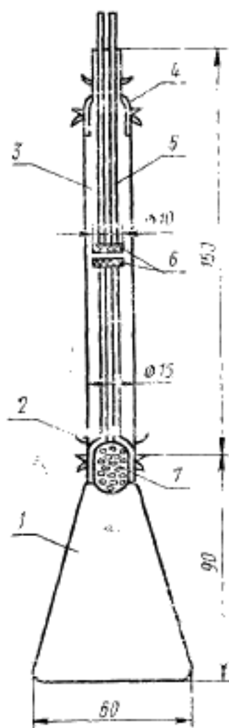
1—колба; 2—пробка; 3—кожух стеклянный; 4—оробка; 5—труб- ка; 6—шлифт; 7—тампон ватный
