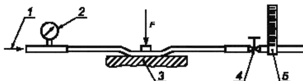
а) Схема испытаний
