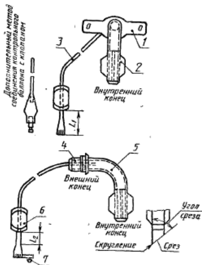
1—фланец; 2—манжета; 3—трубка для раздувания; 4—15-мм диаметровой конический штуцер в соответствии с ГОСТ Р 5—наружная трубка; 6—контрольный баллон; 7—запирающее устройство
