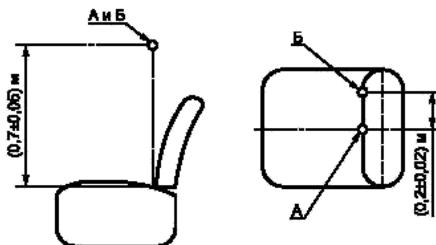
Рисунок 1 — Положение микрофона относительно сиденья
