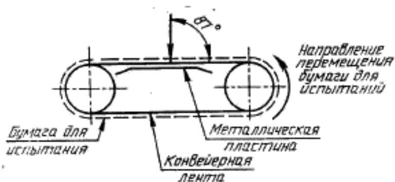
Рисунок 1 — Схема испытательного устройства
