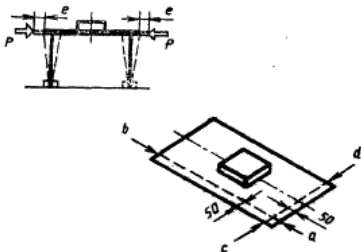
P — нагрузки; e — деформация; a, b, c, d — точки приложения нагрузки
