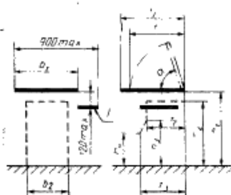
1—полка для чертежных и рисовальных принадлежностей
