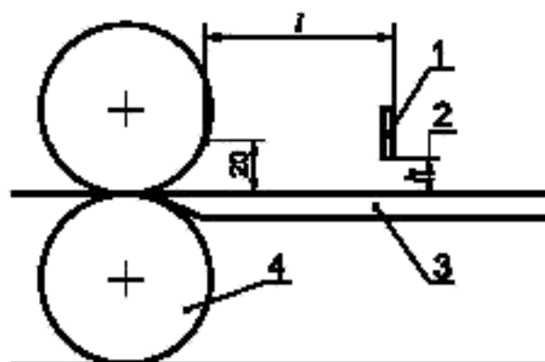
l — барьер; 2 — загрузочное отверстие; 3 — загрузочный стол; 4 — каток
