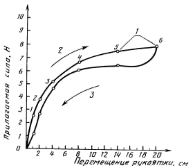
Диаграмма полного закрытого и открытого цикла
