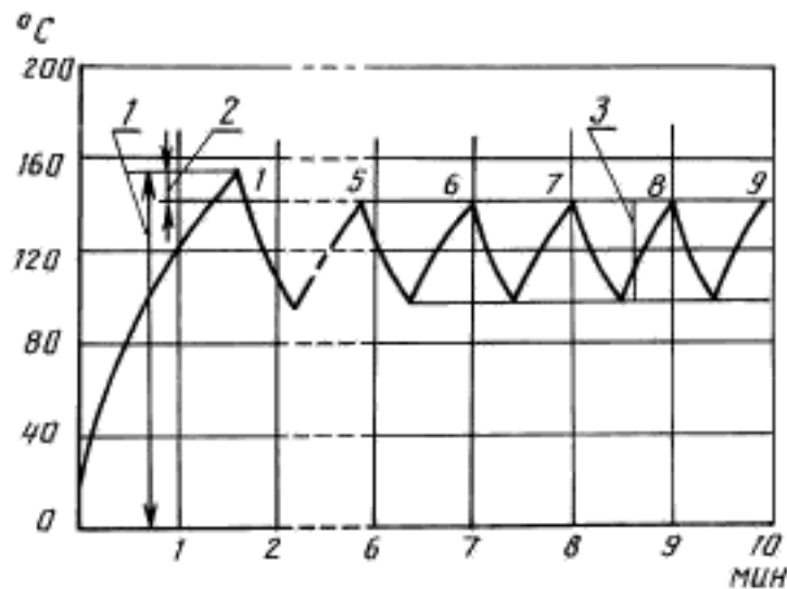
Диаграмма изменения температуры
