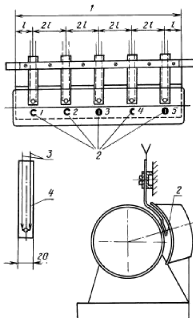
1 — длина башмака; 2 — измерительные точки; 3 — соединение термопар; 4 — лист политетрафторэтилена ( тефлона )
