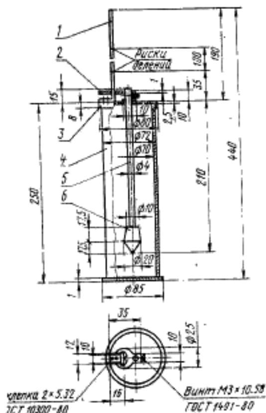
1—шкала; 2—ограничитель; 3—крышка; 4—цилиндр; 5—стержень; 6—груз.
