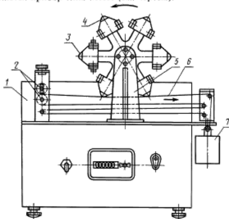
1 — станция; 2 — тянущие валики; 3 — испытуемый образец; 4 — призма; 5 — стойка; 6 — истирающая лента; 7 — груз
