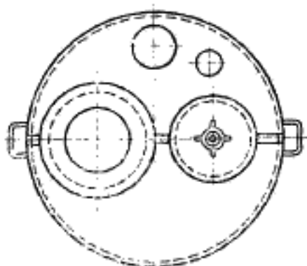
1 — водяная баня; 2 — U-образная трубка; 3 — прижимное кольцо; 4 — манометр; 5 — термометр
