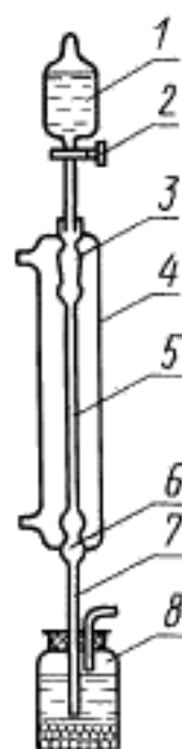
Капиллярный вискозиметр
