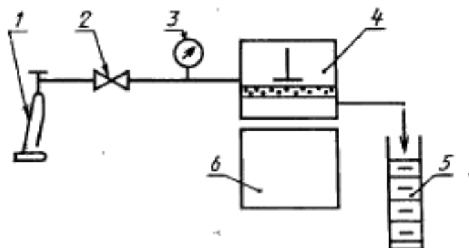
1—баллон со сжатым воздухом или азотом; 2—регулятор давления; 3—манометр; 4—ячейка; 5—медный цилиндр; 6—магнитная мешалка.
